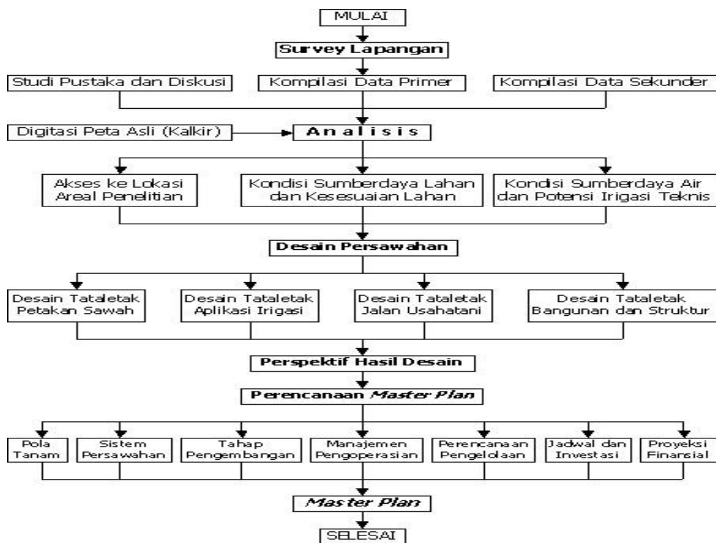
Gambar 1. Diagram skematik desain persawahan dan master plan “Rice Estate Labura” di Desa Ujung Padang, Aek Natas, Labura, Sumut
